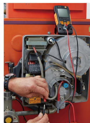
电流测量
