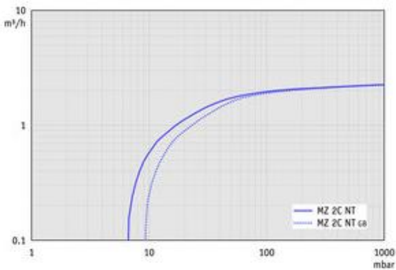
MZ 2C NT - 60 Hz下的抽速曲线
