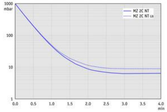
MZ 2C NT - 60 Hz下的抽气曲线 (10升容积)
