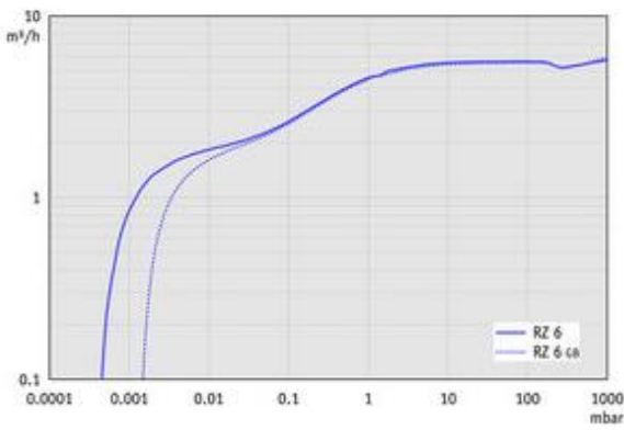
RZ 6 - 60 Hz下的抽速曲线
