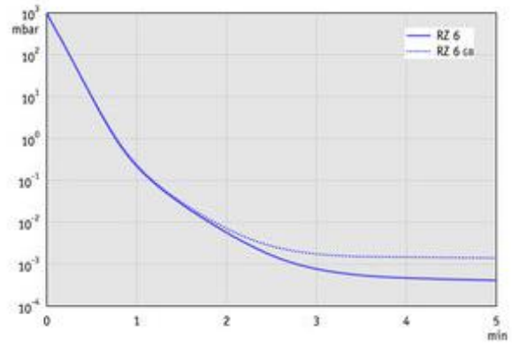
RZ 6 - 60 Hz下的抽气曲线 (10升容积)
