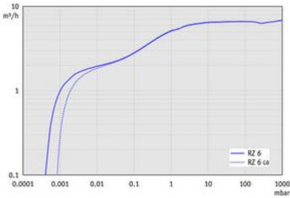
RZ 6 - 60 Hz下的抽速曲线
