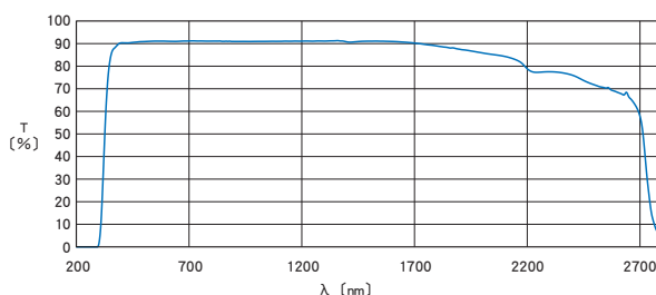
透射率波长特性(参考数据) T: 透射率
