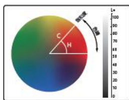
CIE L^*c^*h 色空间
