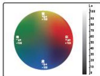
CIE L^*a^*b 色空间
