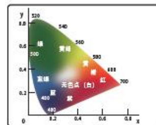
Yxy 色空间
