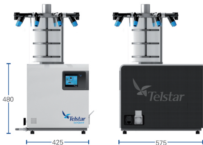
尺寸 (mm)
