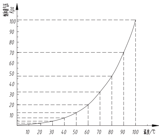
水的饱和蒸汽压曲线图
