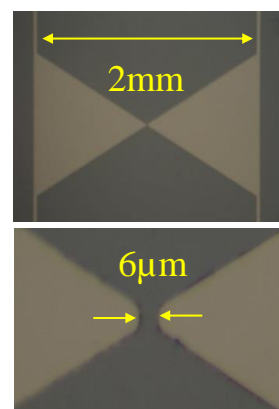
腰隙型
