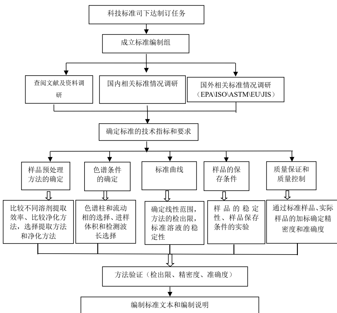
图 1 标准制定的技术路线图
