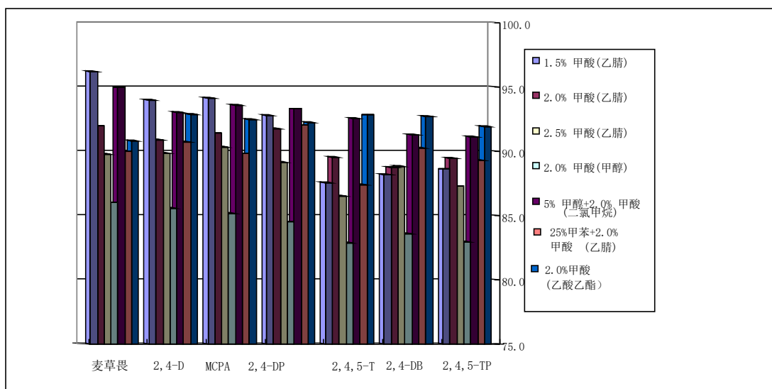
图 45 洗脱溶剂的选择
