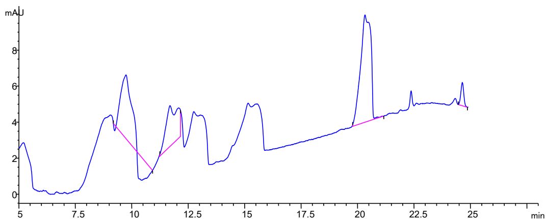
图 22 pH=4.95 的色谱图
