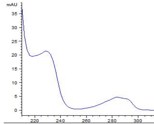
图 25 2,4-D 的吸收光谱图
