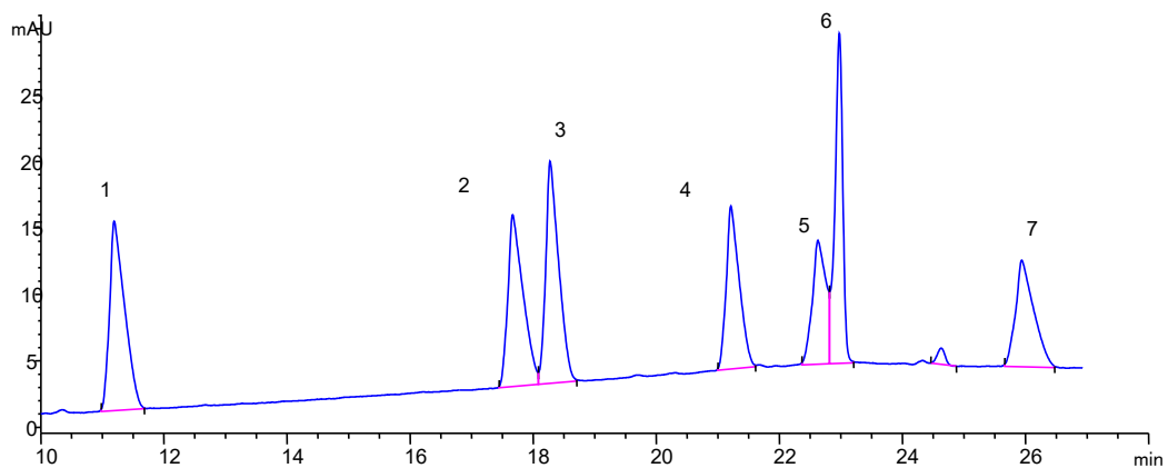
图 20 pH=3.24 的色谱图
