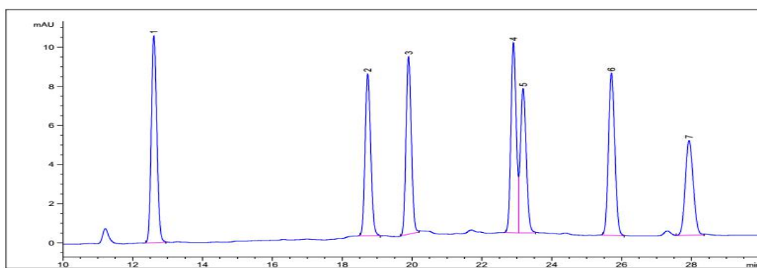
图 34 35°C的色谱图
