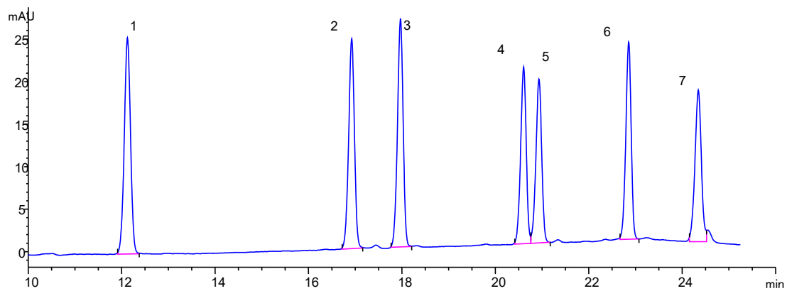
图 16 pH=2.57 的色谱图
