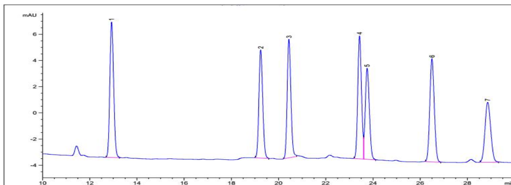
图 33 30°C的色谱图
