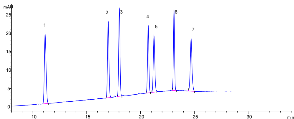
图 36 甲醇+水（2+3）配制 1.00 mg/L 标准溶液的色谱图
