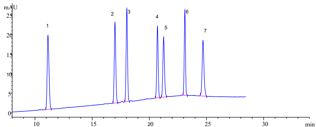
图 46 7 种苯氧羧酸类农药的洗脱曲线
