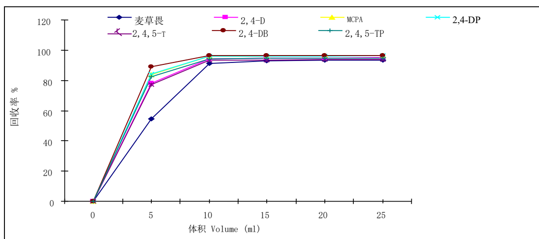
图 46 7 种苯氧羧酸类农药的洗脱曲线
