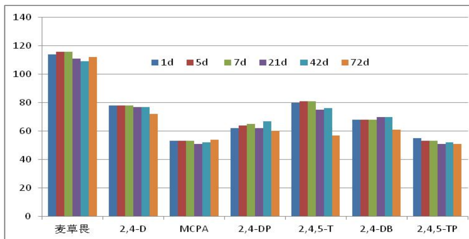
图 7 黄河入海口沉积物中 0.400 mg/L 7 种苯氧羧酸类农药提取净化液的稳定性
