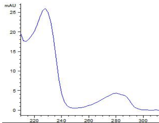
图 26 MCPA 吸收光谱图
