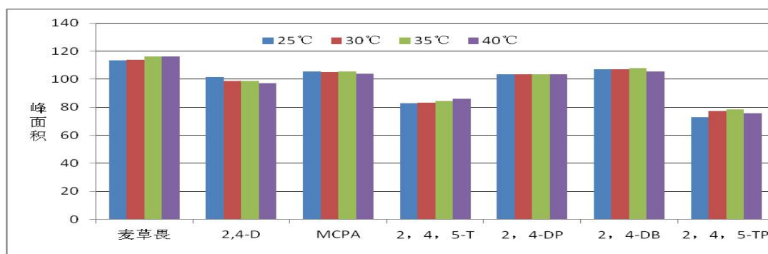
图 31 柱温对峰面积的影响
