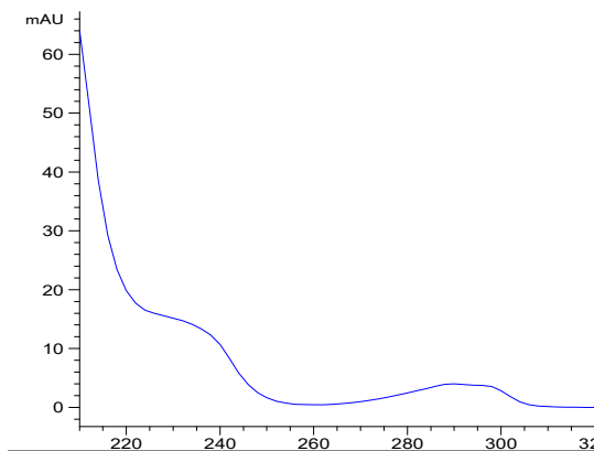
图 28 2,4,5-T 的吸收光谱图
