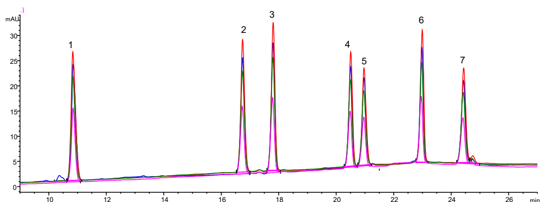
1—麦草畏，2—2,4-D，3—MCPA，4—2,4-DP，5—2,4,5-T，6—2,4-DB，7—2,4,5-TP
