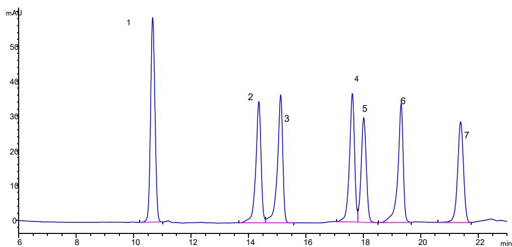
图10 C 18 柱 (150 mm×4.6 mm, 2.7 μm) 分离 7 种苯氧羧酸类农药的色谱图
