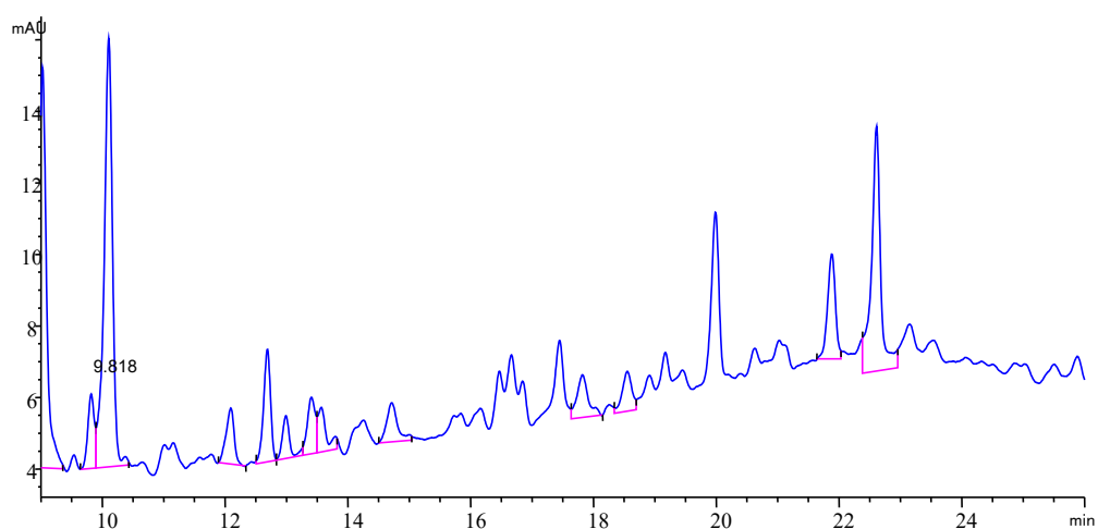
图 48 NH 2 -SPE 净化大沽河土壤样品中 7 种苯氧羧酸类农药加标的色谱图
