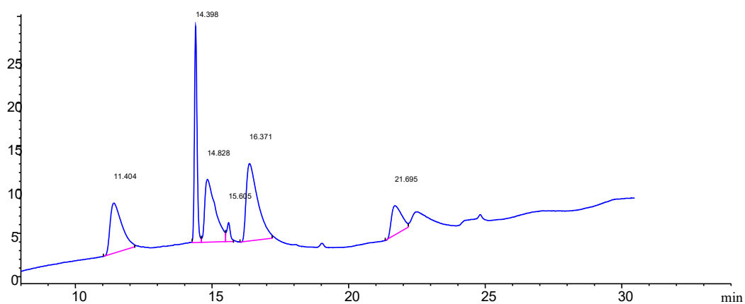
图10 C 18 柱 (150 mm×4.6 mm, 2.7 μm) 分离 7 种苯氧羧酸类农药的色谱图
