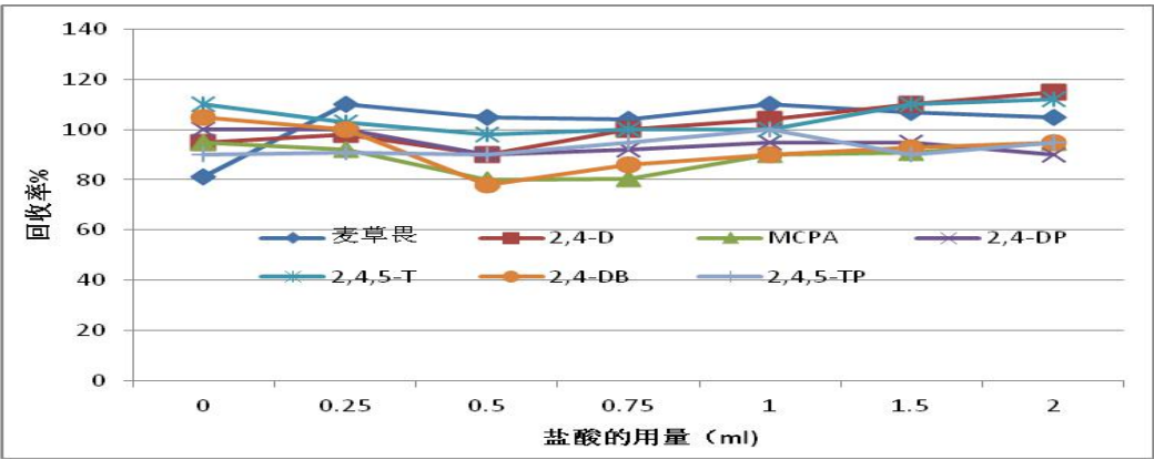
图 40 不同体积的盐酸对测定 7 种苯氧羧酸类农药回收率的影响
