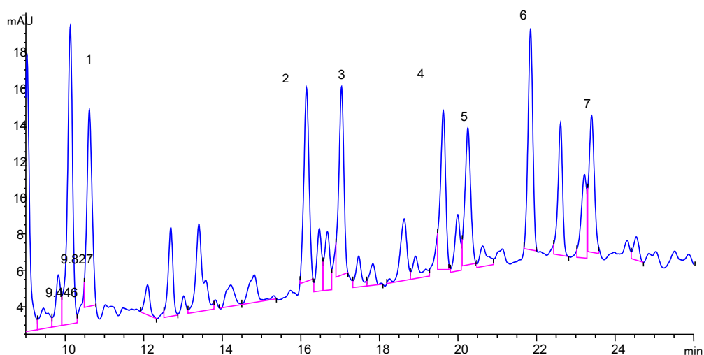
图 48 NH 2 -SPE 净化大沽河土壤样品中 7 种苯氧羧酸类农药加标的色谱图
