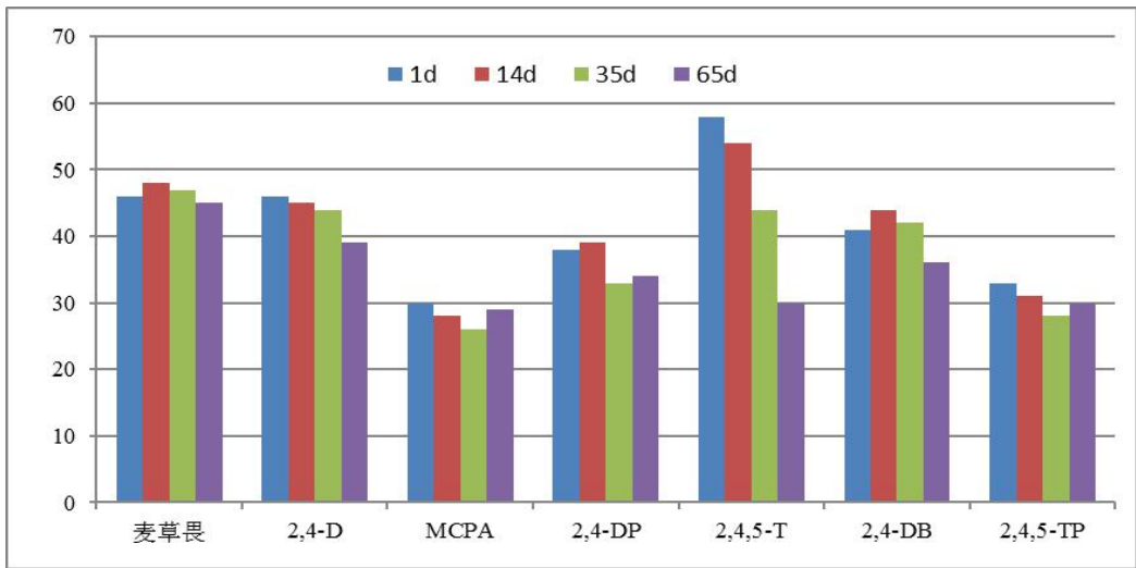
图 6 青岛潮棕土中 0.200 mg/L 7 种苯氧羧酸类农药提取净化液的稳定性
