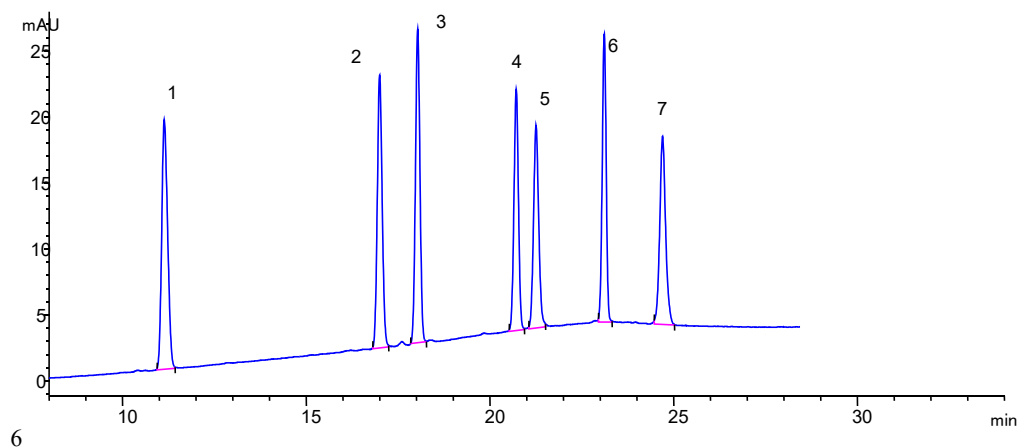
图9 C 8 柱 (150 mm×4.6 mm, 2.7 μm) 分离 7 种苯氧羧酸类农药的色谱图
