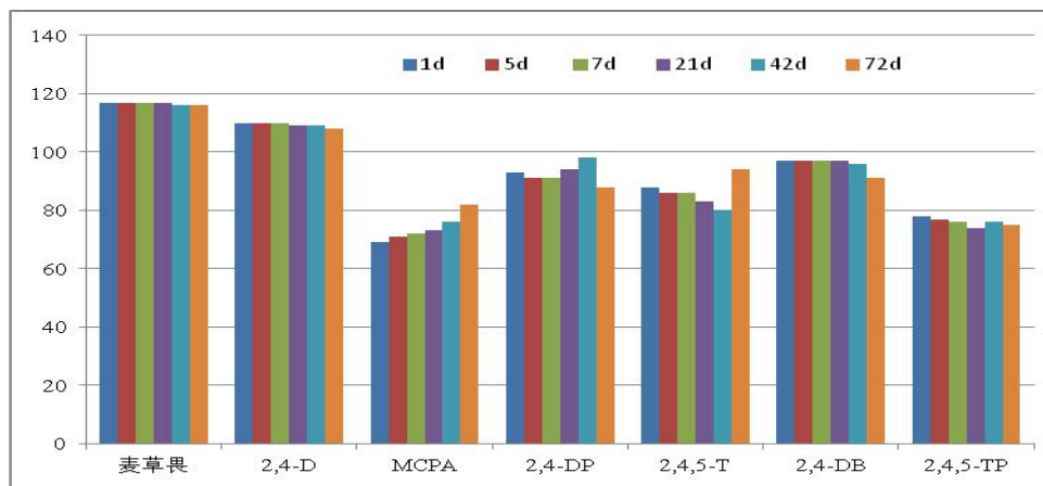
图 3 0.400 mg/L 的 7 种苯氧羧酸类农药的工作溶液的稳定性
