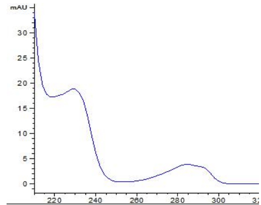
图 27 2,4-DP 的吸收光谱图
