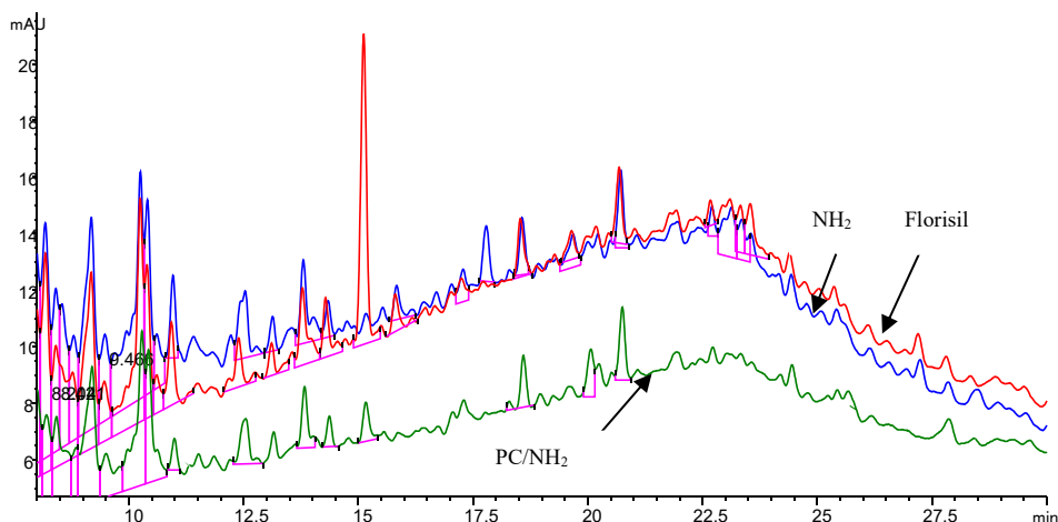
图 44 NH 2 柱、Florisil 柱、PC/NH 2 柱净化农科院花园土壤本底的色谱图
