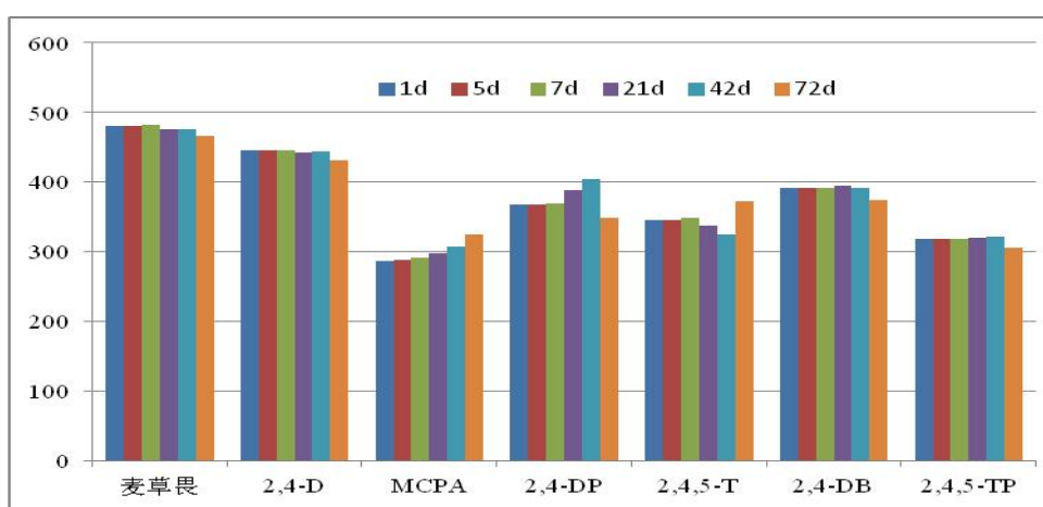
图 5 2.00 mg/L 的 7 种苯氧羧酸类农药的工作溶液的稳定性
