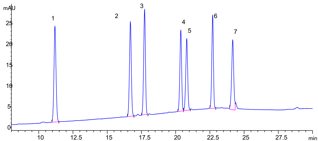
图 17 pH=2.94 的色谱图
