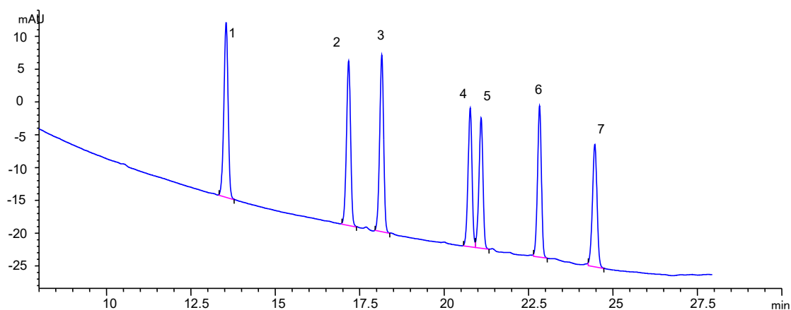
图 15 pH=2.28 的色谱图
