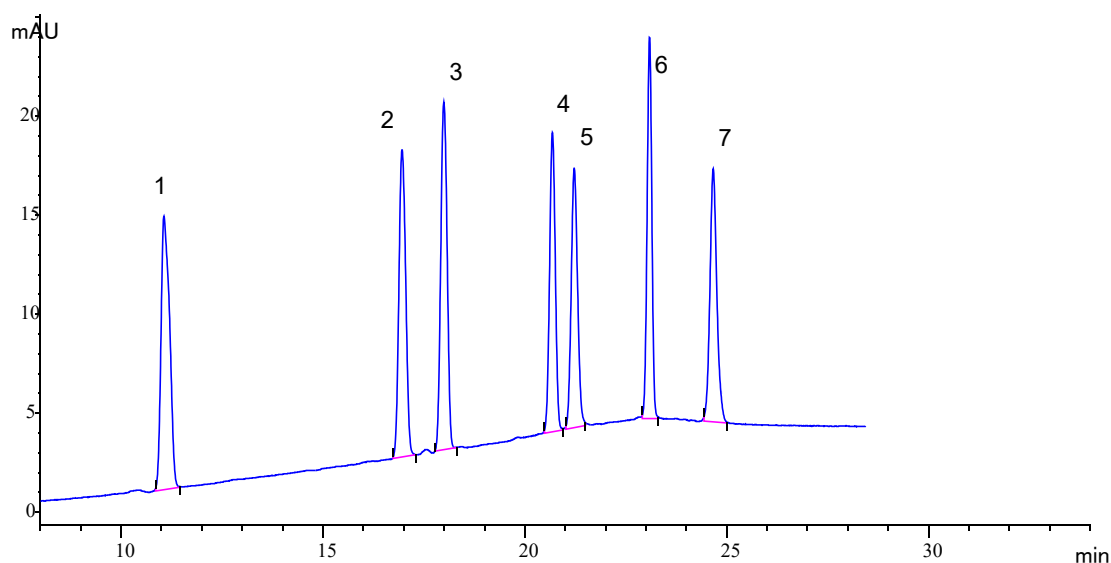
图 37 甲醇+水（3+2）配制 1.00 mg/L 标准溶液的色谱图
