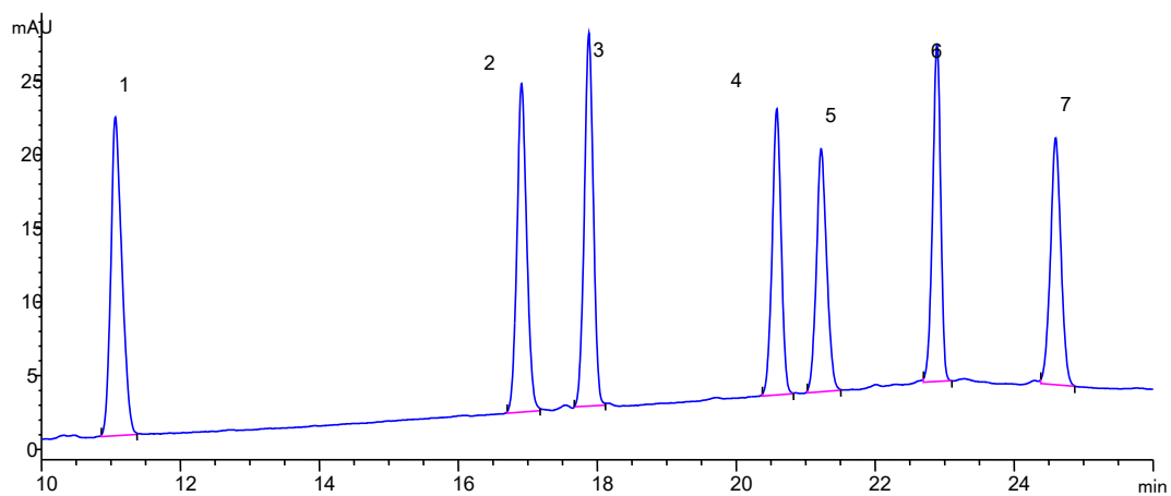
图 19 pH=3.10 的色谱图
