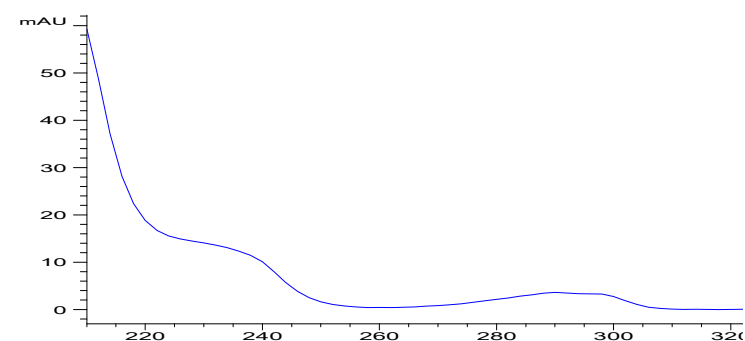
图 30 2,4,5-TP 的吸收光谱图
