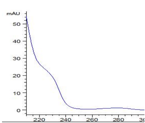
图 24 麦草畏的吸收光谱图
