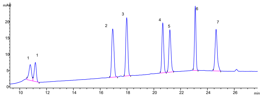
1—麦草畏, 2—2,4-D, 3—MCPA, 4—2,4-DP, 5—2,4,5-T, 6—2,4-DB, 7—2,4,5-TP
