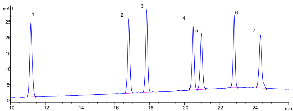
图 16 pH=2.57 的色谱图
