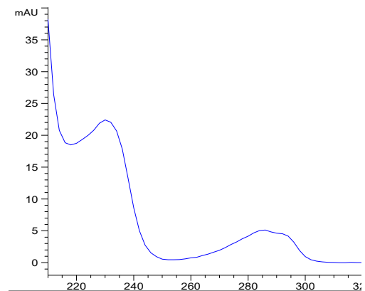
图 29 2,4-DB 的吸收光谱图
