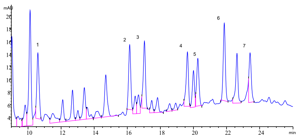
图 49 NH 2 -SPE 净化大沽河土壤样品的色谱图
