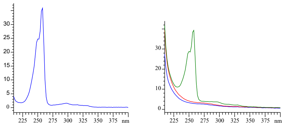
图 51 大沽河土壤样品中干扰物的光谱图
