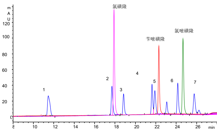
图 51 氯磺隆、苄嘧磺隆和氯嘧磺隆对测定 7 种苯氧羧酸类农药的影响
