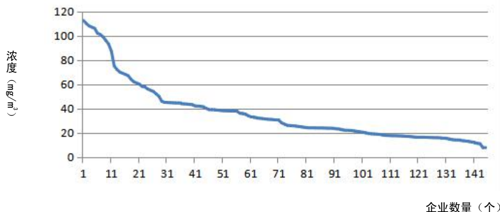
图 5-6 电弧炉颗粒物排放浓度统计 (mg/m 3 )
