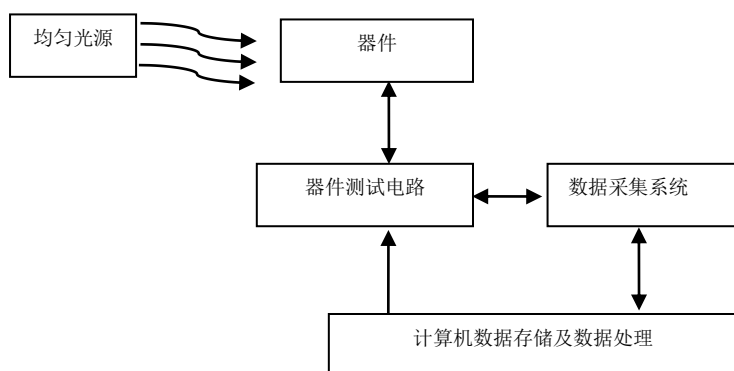
图 08-1 光响应非均匀性测试原理框图
