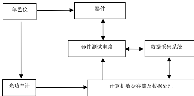
图 10-2 相对光谱响应测试原理框图
