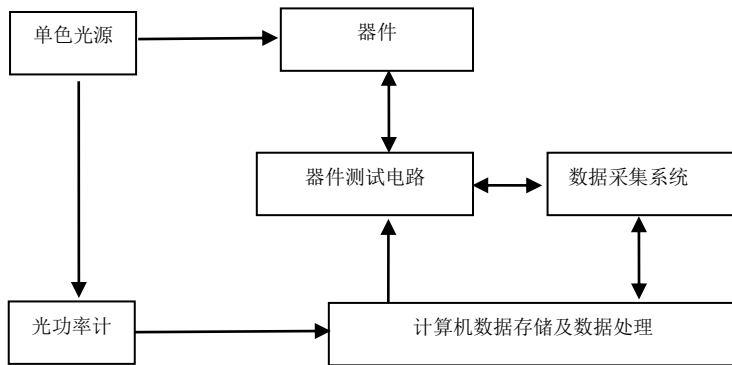
图 10-1 单色光响应率测试原理框图
