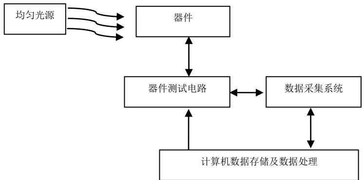
图 07-1 缺陷测试原理框图
