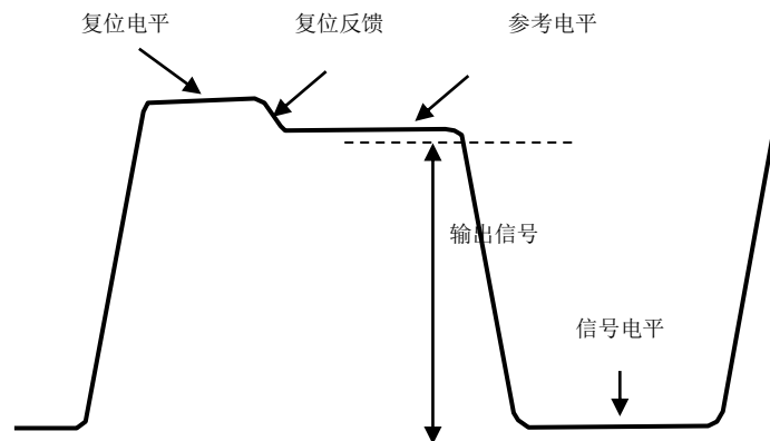
图3 器件像元信号理想输出波形
